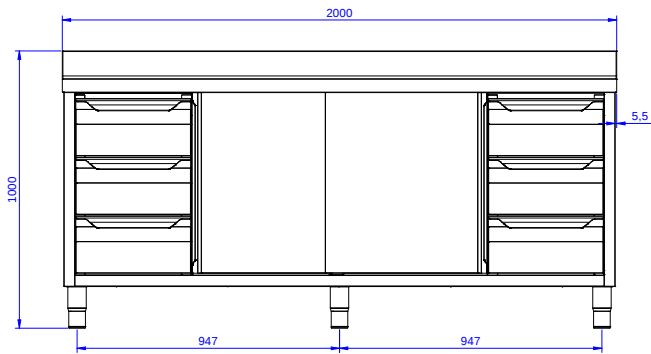
Alzado
